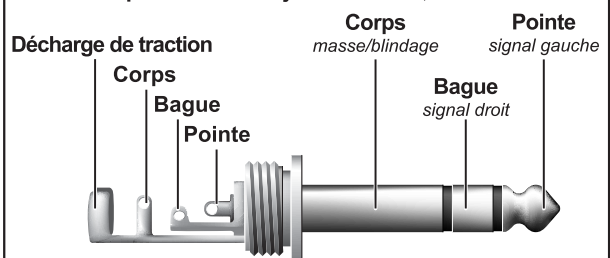
Fig. 4.4 : Jack stéréo pour casque
